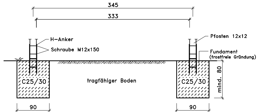
Schnitt A-A
