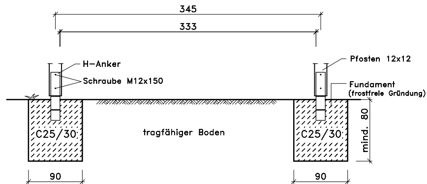
Schnitt B-B
