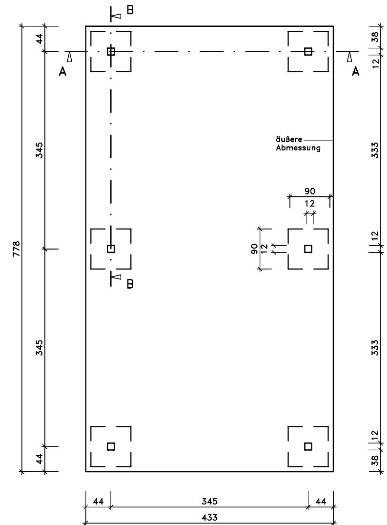
Grundriß
