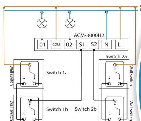
Technisch installatie schema van de ACM-3000H2
