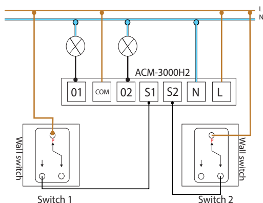
Technisch installatie schema van de ACM-3000H2
