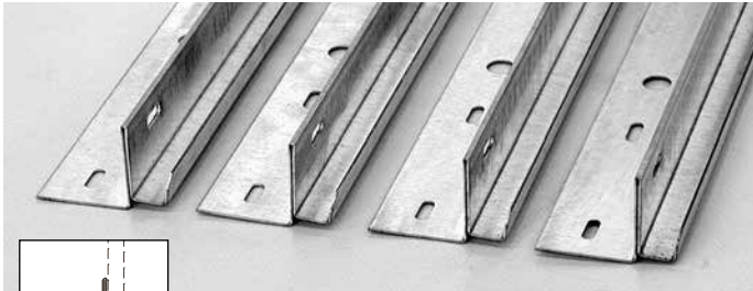
Bodenprofil (verzinkt) (A) bottom frame (galvanised) (A) profil de sol (galvanisé) (A) profilo a pavimento (zincato) (A)
