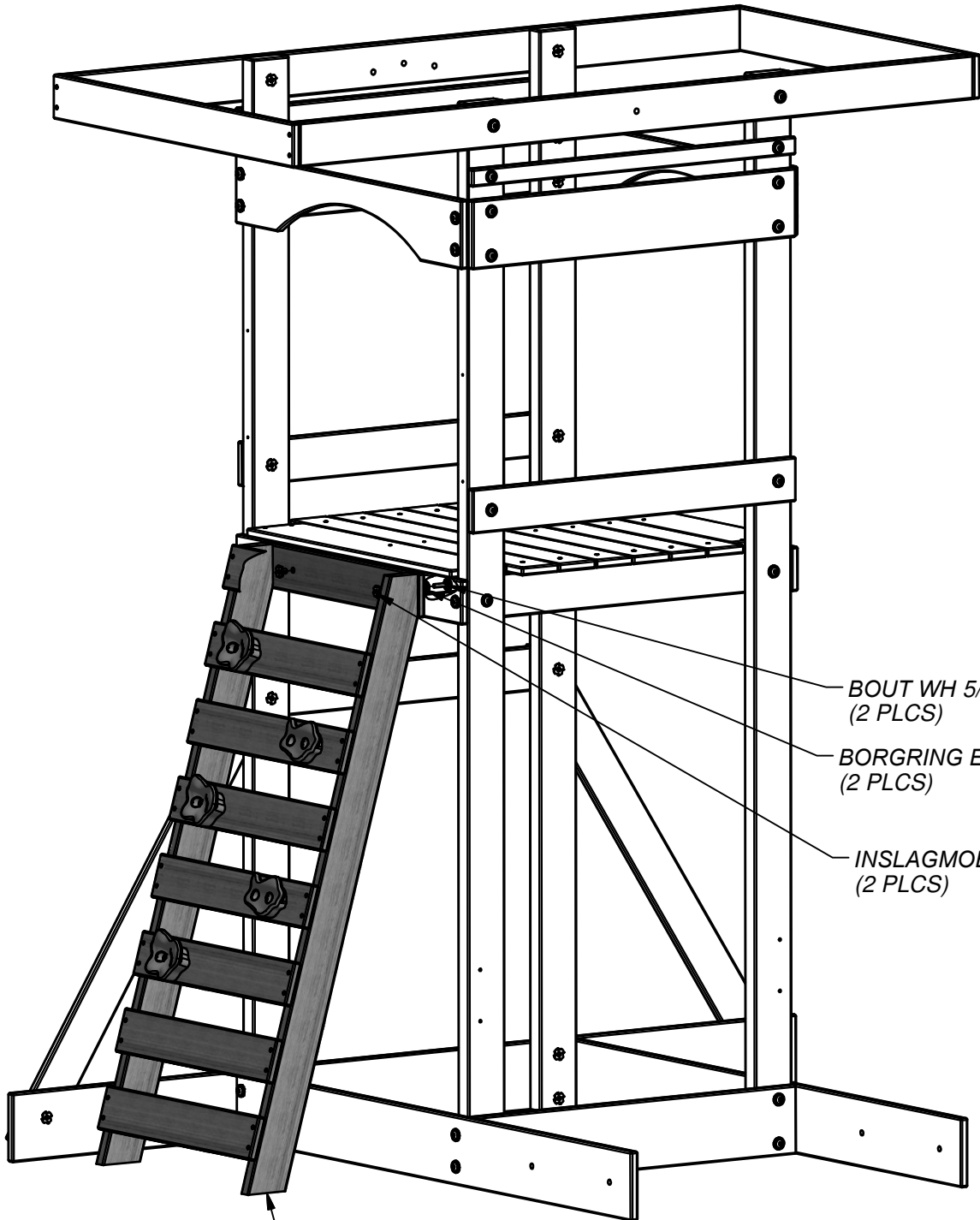
STEEN LADDER MONTAGE
