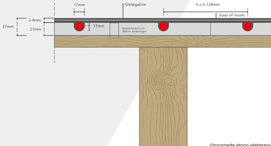
Doorsnede Mono gietmassa
