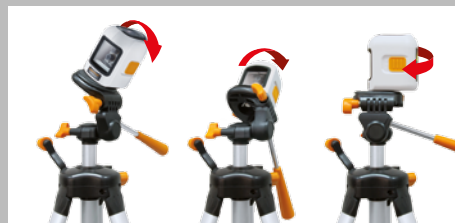
3-weg-statiefkop
