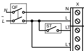
MIN SVORKOVNICE PRO 5 KONTAKTŮ
