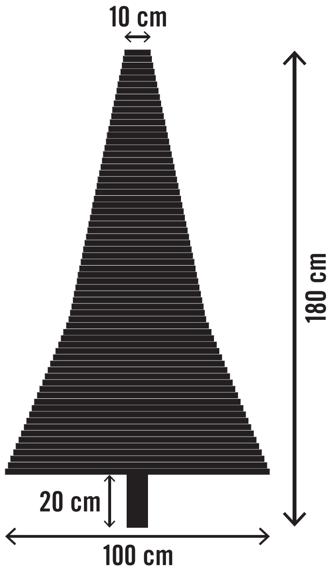
Zijaanzicht
