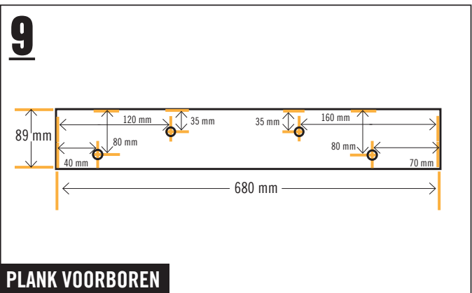
LEGPLANK VOORBOREN EN BEVESTIGEN
